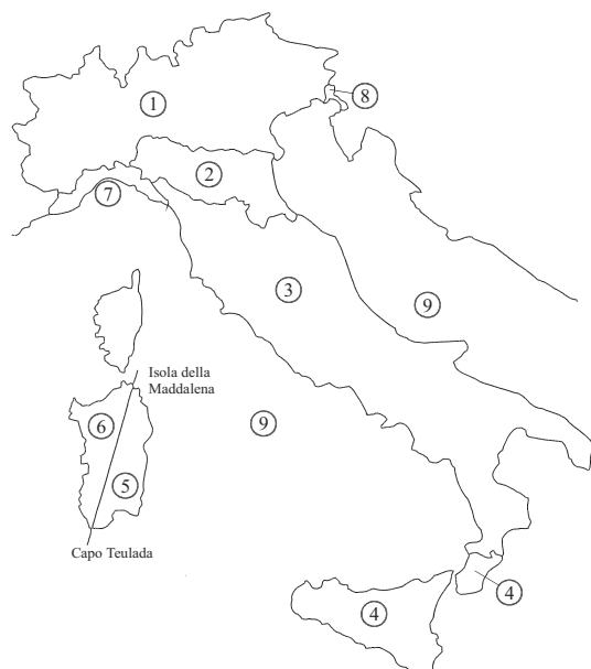
Figura 3.3.1 – Mappa per la macrozonazione per l'azione del vento
